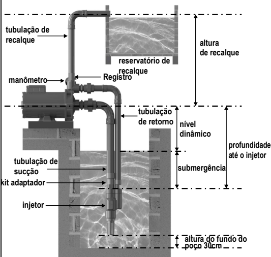
Fig. 02 - Instalação injetoras
