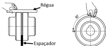
Fig. 08 – Alinhamento com régua e espaçador
