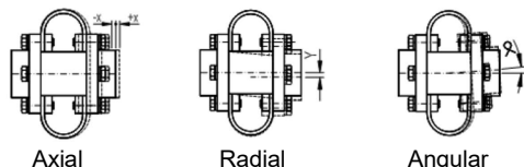
Fig. 07 – Tipos de desalinhamentos
