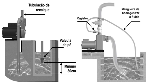
Fig. 03 - Instalação Autoaspirantes
