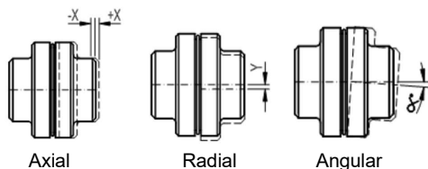
Fig. 06 – Tipos de desalinhamentos
