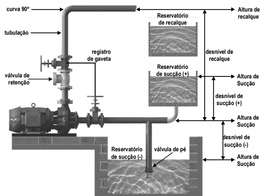
Fig. 01 - Instalação com válvula de pé ou afogada
